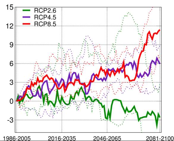
Сл. 8 Промени во последователни сушни денови (во денови) за последователни 20-годишни периоди почнувајќи од 1986-2005 до 2081-2100, во однос на периодот 1986-2005, за сценаријата RCP2.6, RCP4.5 и RCP8.5. Полните линии се средна вредност на збир од повеќе избрани модели, а точкестите линии се збирен опсег од 25-тиот до 75-тиот перцентил.
