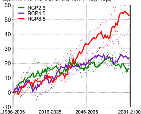
Сл. 9 Промени во должината на вегетациониот период (во денови) за последователни 20-годишни периоди почнувајќи од 1986-2005 до 2081-2100, во однос на периодот 1986-2005, за сценаријата RCP2.6, RCP4.5 и RCP8.5. Полните линии се средна вредност на збир од повеќе избрани модели, а точкестите линии се збирен опсег од 25-тиот до 75-тиот перцентил.
