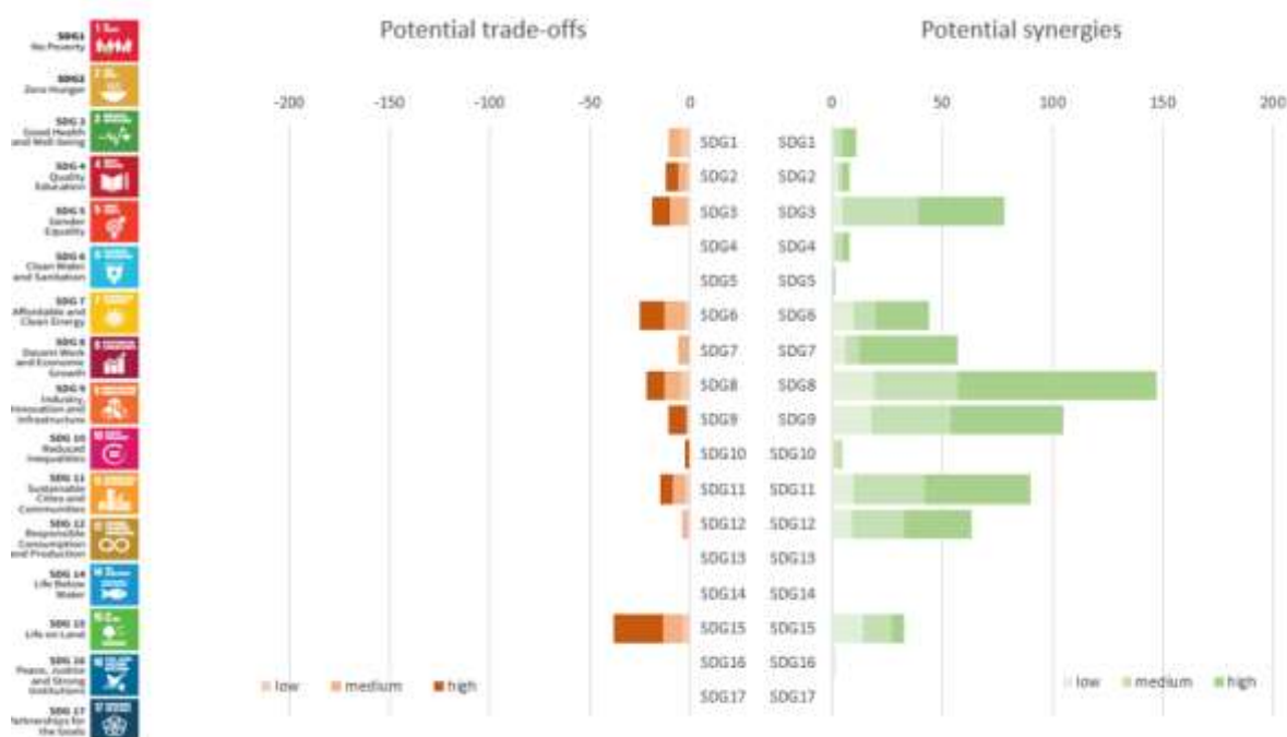
Слика 3. Електрична и топлинска енергија, Транспорт и Згради – синергии и компромиси со ЦОР
